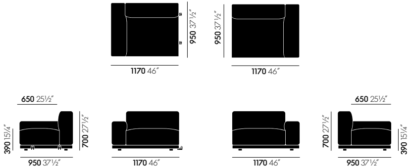
Seitenelement rechts
