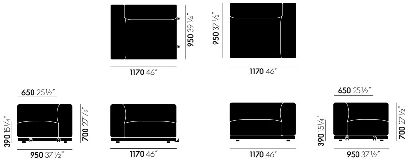
Seitenelement rechts
