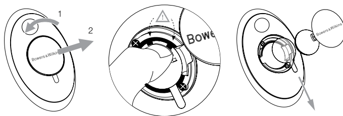
Obrázek 3 Odstranění izolačního krytu A7
